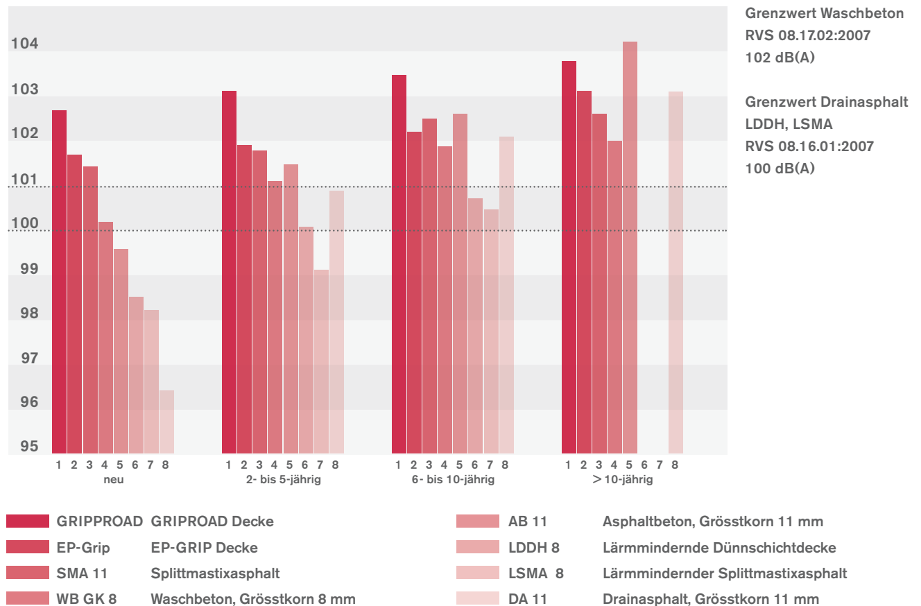
Abbildung 2: Rollgeräuschpegel auf Decken unterschiedlichen Alters [1]
