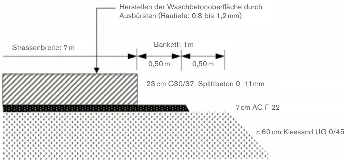
Aufbau des neuen Strassenkörpers
