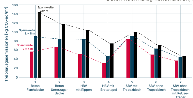
Abbildung: Ökobilanzielles Potential von Stahlbeton- und Verbunddecken-systemen bei verschiedenen Spannweiten. Quelle: Deckensysteme mit Beton nachhaltig konstruieren, ZHAW
