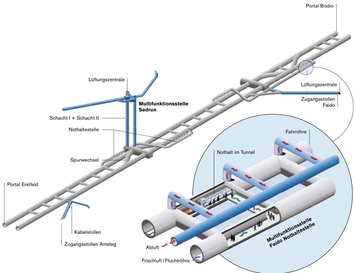
Abbildung 1: Schema Tunnelsystem GBT mit Notthaltestelle und Lüftung © AlpTransit Gotthard AG
