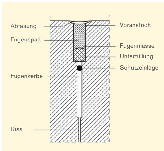
Scheinfuge
