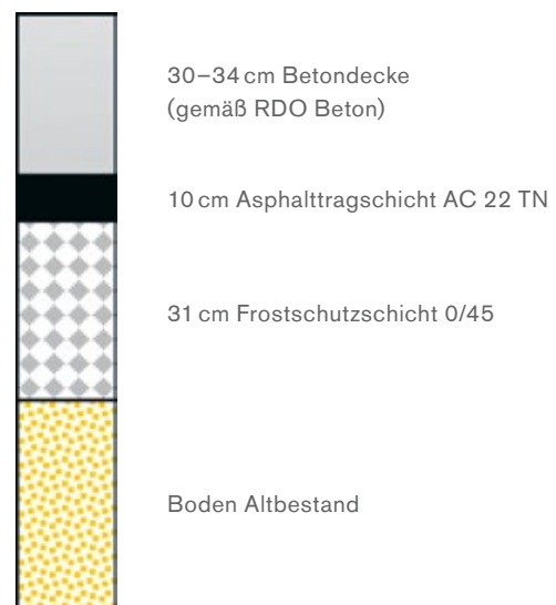
Aufbau Gesamtquerschnitt ZOB Singen
