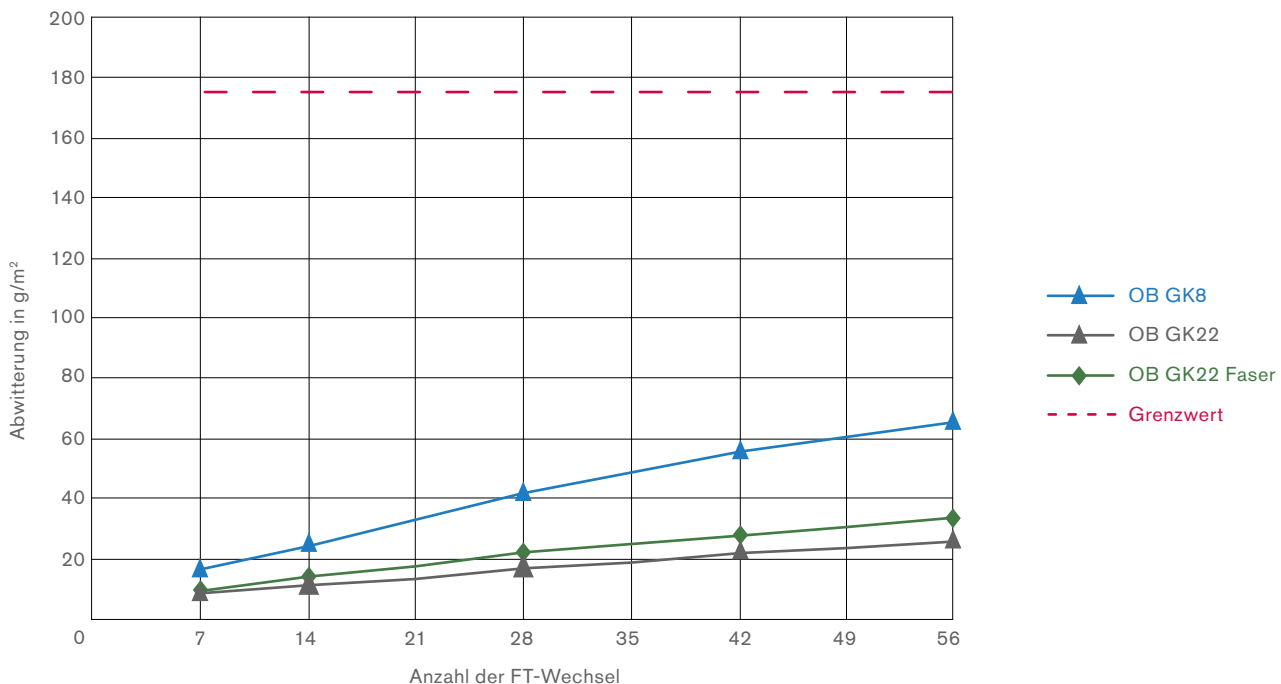
Frost-Taumittel-Prüfung der Proben (Nachweise der Expositions-kategorie XF4)
